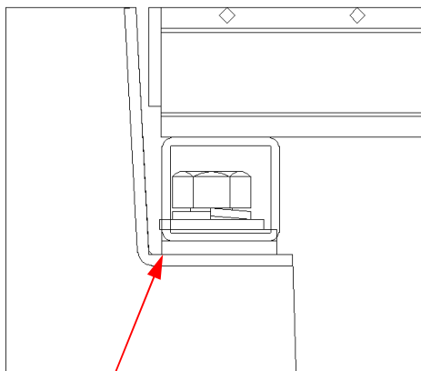
アングルありタイプ
