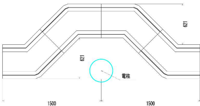
◆電柱よけ施工図
