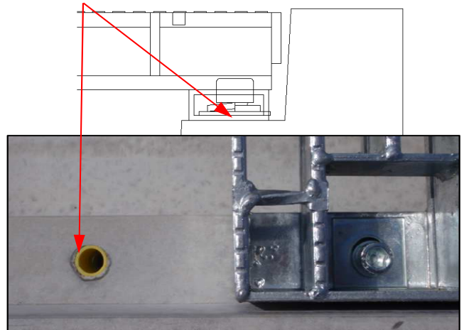
アングルなしタイプ
