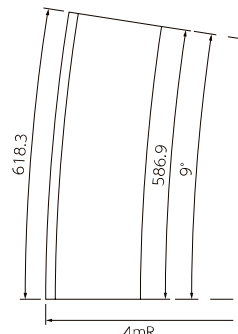
乗入タイプ・横断歩道接続部（片面）4mR （10分割）
