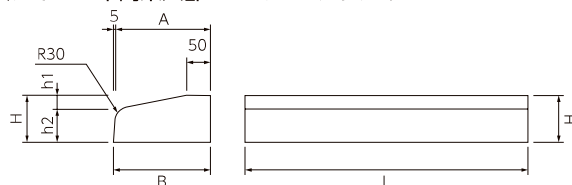
乗入タイプ・車両乗入部 セミフラットタイプ
