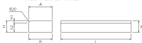
乗入タイプ・車両乗入部 フラットタイプ（両面）
