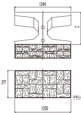
KPB大型ブロック A型 (基本 SL=800、L=1,250)
