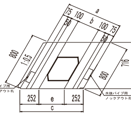
KPB大型ブロック A型 (基本 SL=800、L=1,250)
