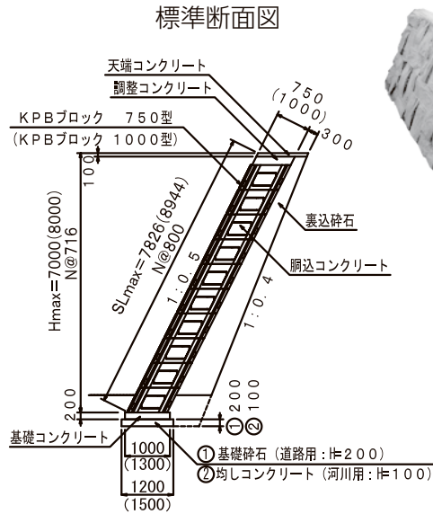
KPB大型ブロック A型 (基本 SL=800、L=1,250)
