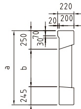
基礎ブロック
