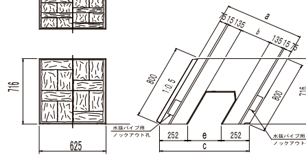
KPB大型ブロック B型 (基本 SL=800、L=625)
