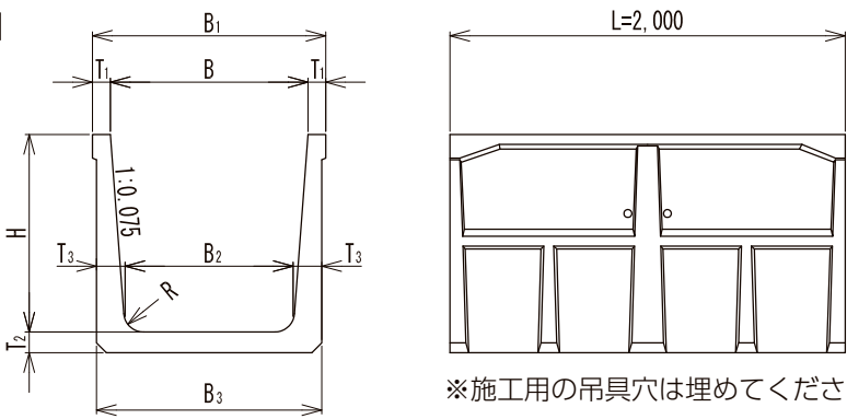
標準図
