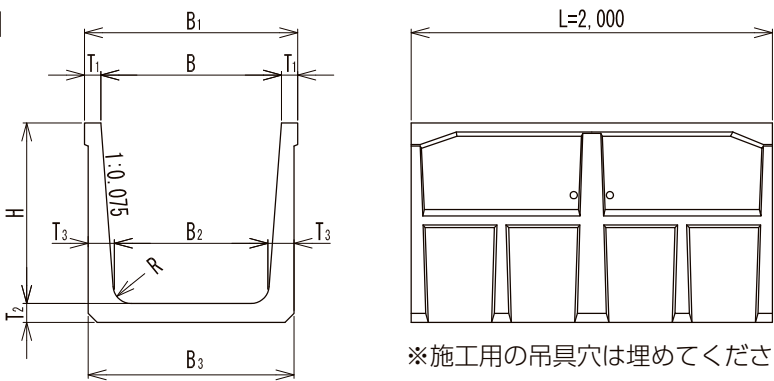
標準図
