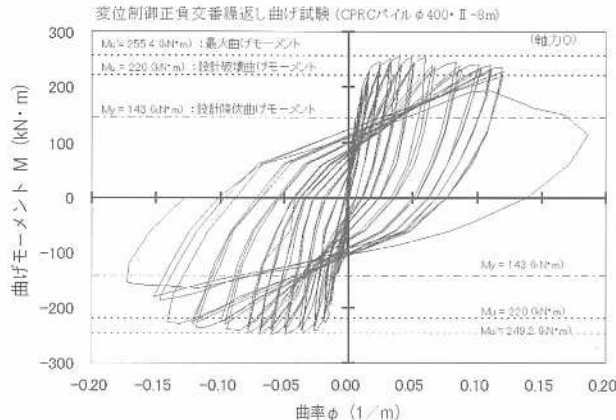
φ400mm (Ⅱ種) 曲げモーメントと曲率の関係
